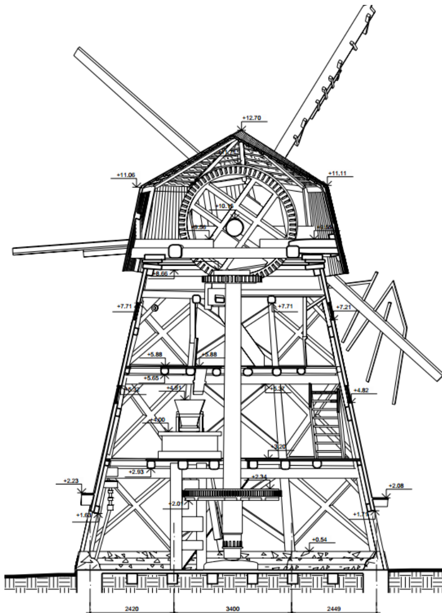
Pjūvis M 1:50 (brėžinio tipas Nr.: 3)
