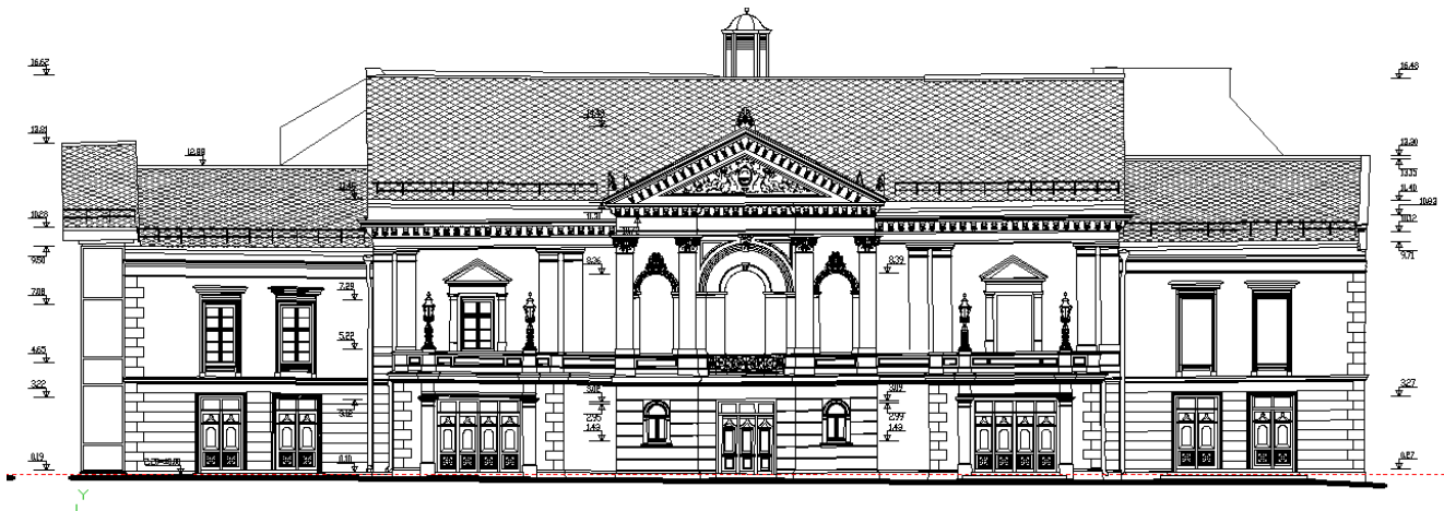
Fasadų išklotinė – kultūros paveldo objektui M 1:50 (brėžinio tipas Nr.: 2)
