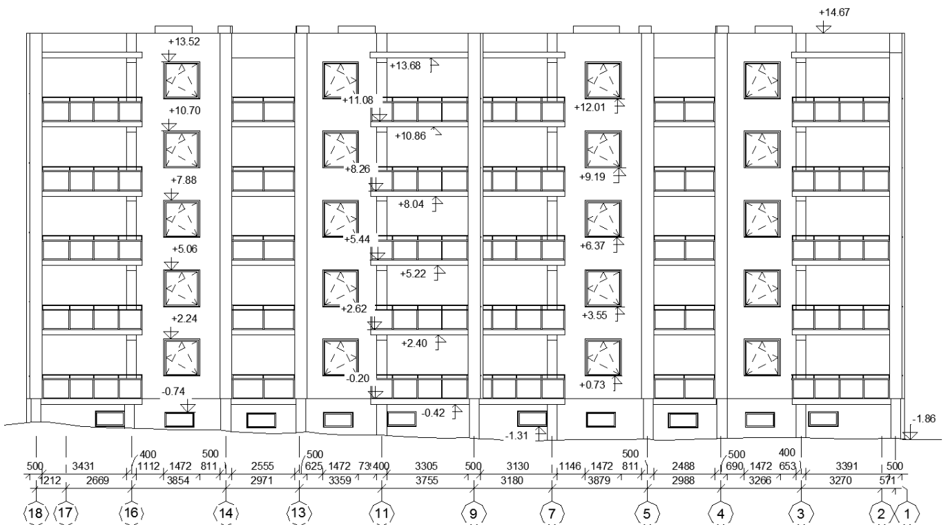
Fasadų išklotinė – renovacijos projektui M 1:100 (brėžinio tipas Nr.: 1)
