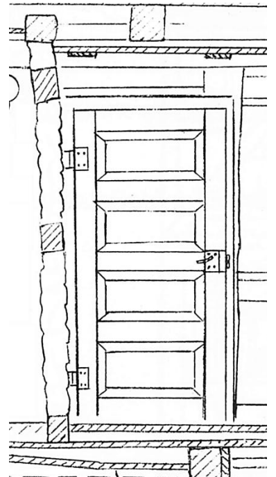
Brėžinio tipas Nr.: 3
