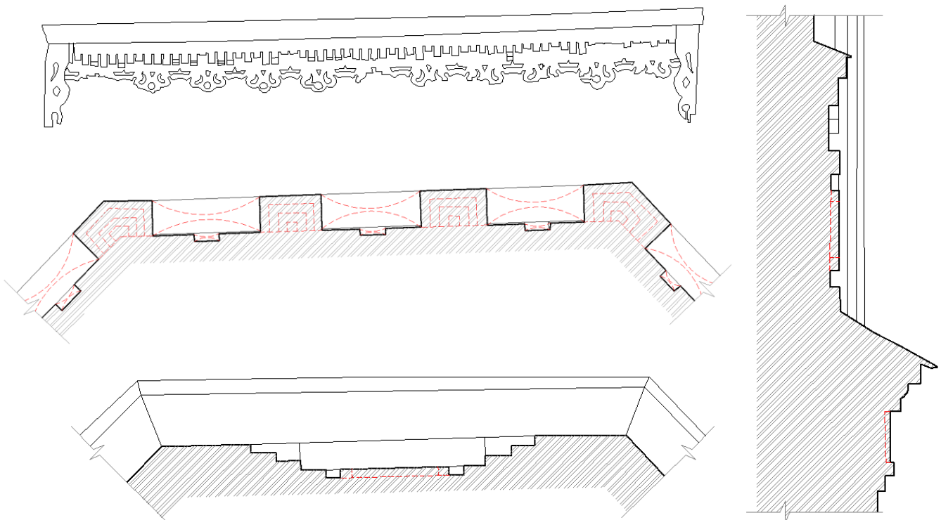
Pjūviai – detalizuotos vietos M 1:10; M 1:25 (brėžinių tipai Nr.: 3-4)
