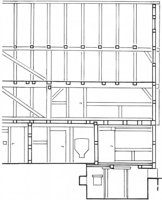
Brėžinio tipas Nr.: 1 M 1:100
