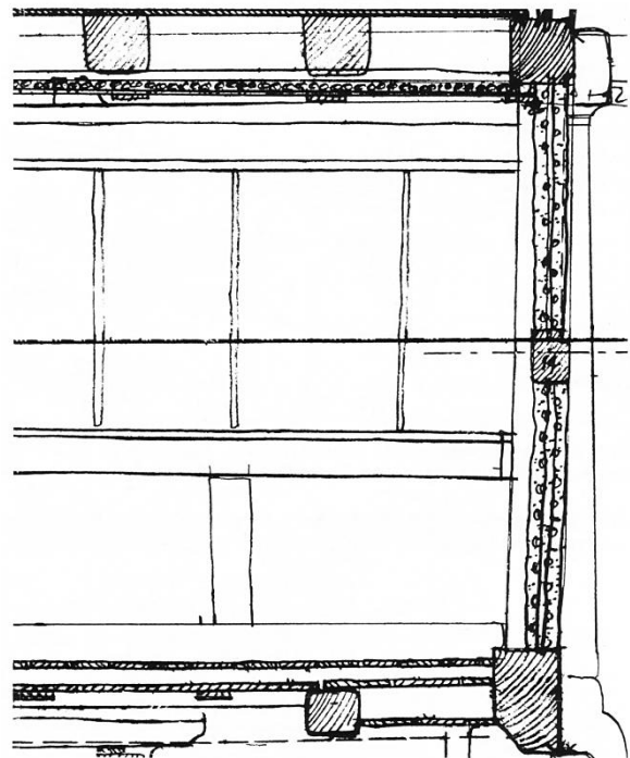
Brėžinio tipas Nr.: 4 M 1:25; 1:10
